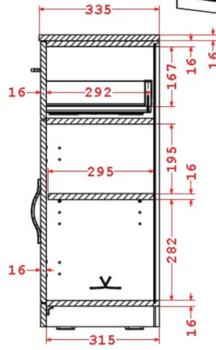
SEZIONE A-A
